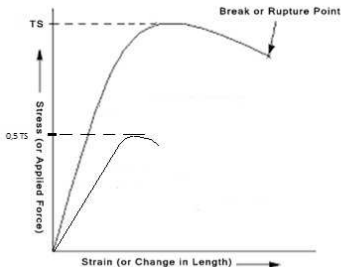
Figura 1: Resistenza alla trazione a seguito di esposizione UV
